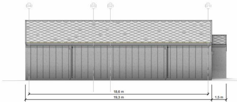
Fasade nord
