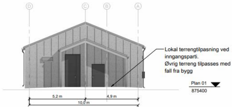
Fasade vest
