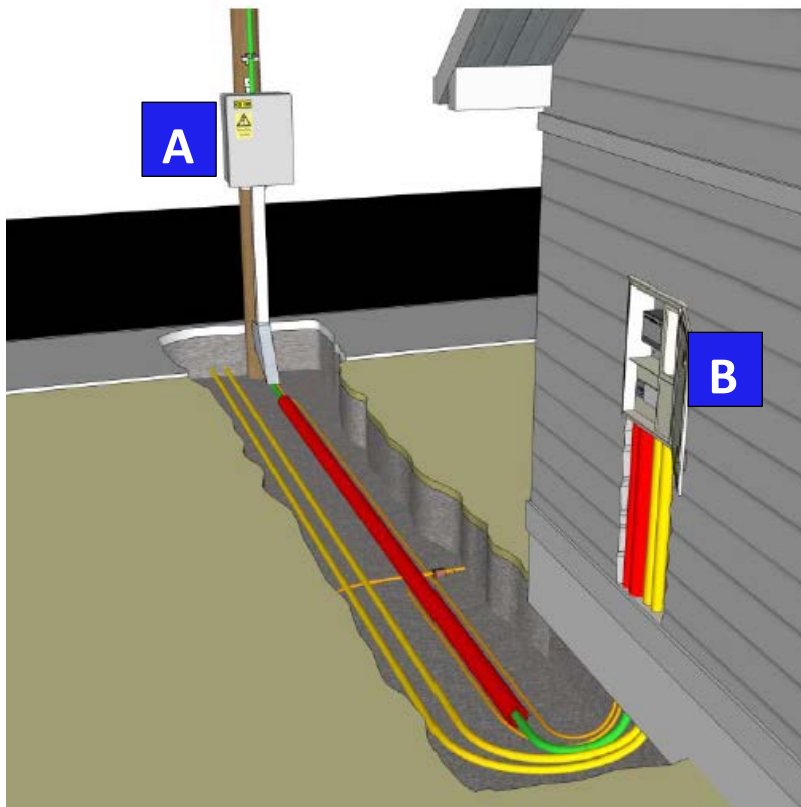
Figur viser stolpeskap som eies av Skagerak Nett (A) og tilknytningsskap som eies av kunde (B). Tilknytningsskapet (B) er her innfelt i vegg hos kunde.
