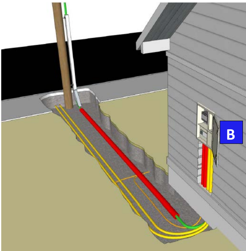
Figur viser at kabel kommer direkte fra luftnett uten å gå via kabelskap. Tilknytningsskapet (B) eies av kunde og er her innfelt i vegg hos kunde.
